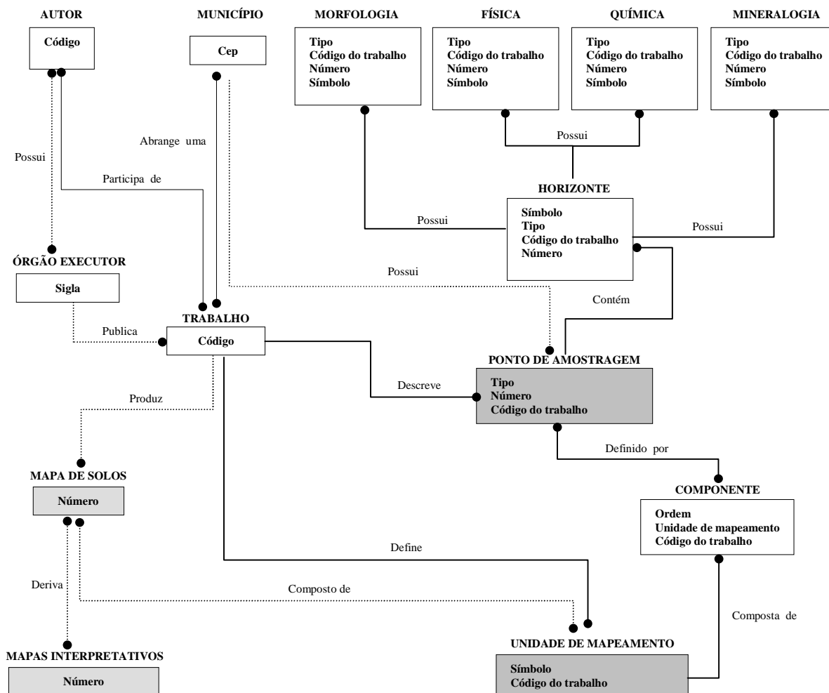
Figura 2. Modelo conceitual simplificado do SigSolos.
