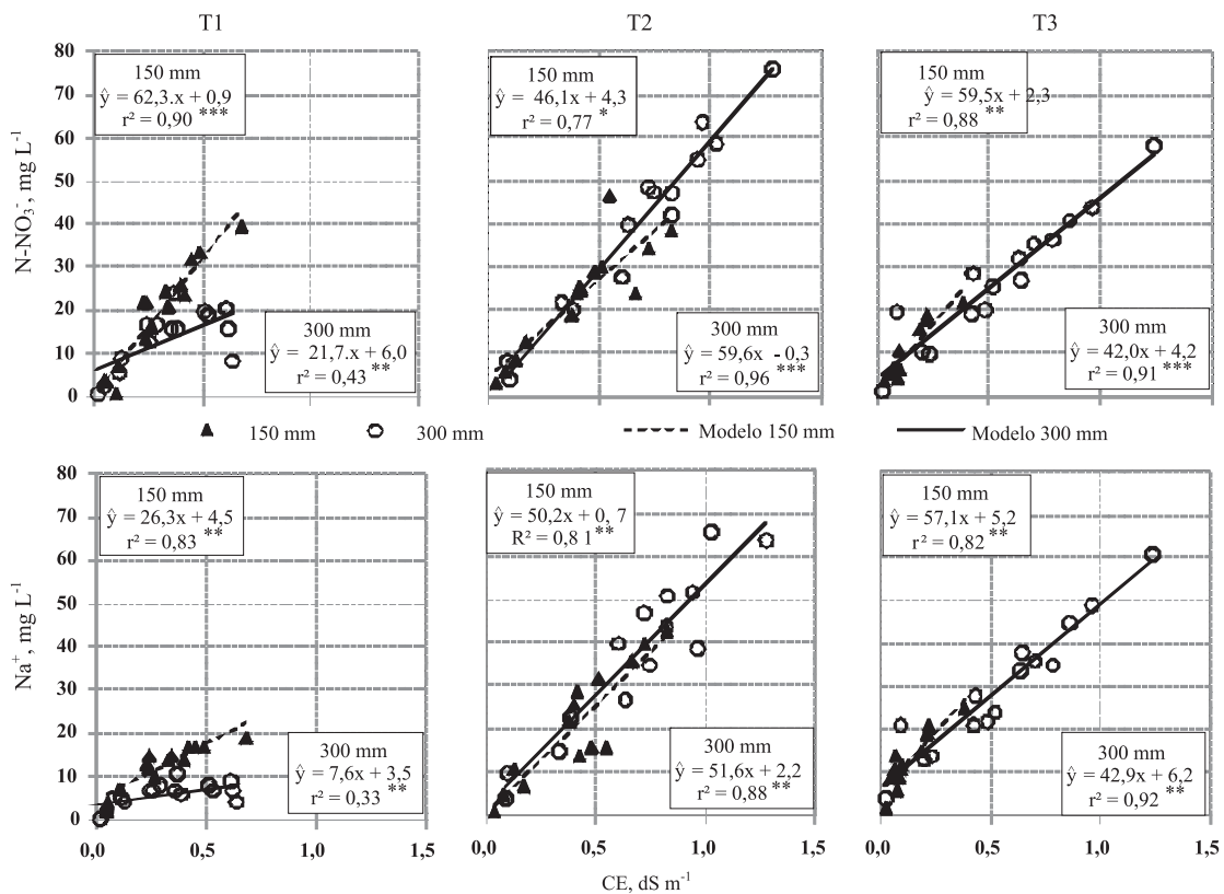
Figura 3. Relação entre \text{Na}^+ , \text{NO}_3^- e condutividade elétrica (CE) na solução do solo após aplicação de 150 e 300 mm de água (T1), de efluente EETE (T2) e de efluente EETE + \text{CaSO}_4 (T3). ** p < 0,01 ; *** p < 0,05 .
