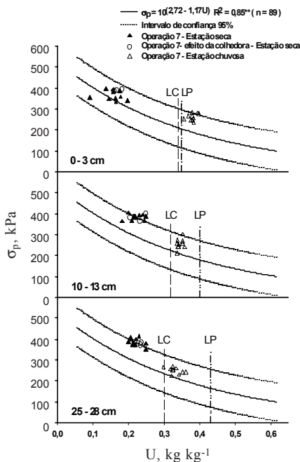
Figura 6. Modelo de capacidade de suporte de carga para o Latossolo Amarelo distrófico típico nas camadas de 0–3, 10–13 e 25–28 cm com seus respectivos limites de contração (LC) e de plasticidade (LP). Os pontos representam as pressões de preconsolidação determinadas após as operações de todos os equipamentos na estação seca e na chuvosa (Operação 7).
