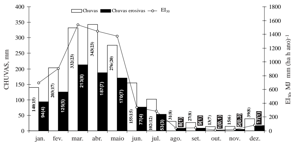
Figura 1. Distribuição de valores médios mensais das chuvas e das chuvas erosivas em relação aos valores médios mensais do índice El_{30} no período de 1962 a 1981, em Fortaleza (CE). Valores entre parêntese indicam o número médio de chuvas abaixo dos quais são indicados os valores médios mensais das chuvas em mm.
