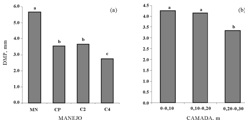
Figura 1. Valores de diâmetro médio ponderado (DMP) de agregados do Latossolo Vermelho caulinitico (LVd) submetido a diferentes manejos (a), utilizando o valor médio da camada de 0-0,30 m, e camadas (b), usando o valor médio de todos os manejos. MN: mata nativa; CP: cana planta; C2: cana soca de segundo ano; C4: cana soca de quarto ano. Médias seguidas de mesma letra não diferem estatisticamente pelo teste de Tukey a 5 %.
