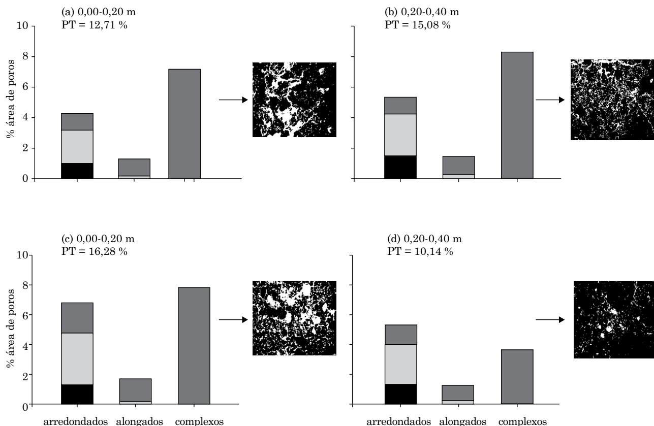
Figura 1. Forma e tamanho de poros quantificados pelas imagens 2D (poros em branco, fase sólida em preto) e porosidade total (PT) em duas profundidades de um Latossolo Vermelho distroférico típico manejado com semeadura direta [SD: (a), (b)] ou preparo convencional [PC: (c), (d)]. Poros: ■ Pequeno (0,00156-0,0156 mm 2 ); ■ Médio (0,0156-0,156 mm 2 ); ■ Grande (>0,156 mm 2 ). (a) SD 0,00-0,20 m; (b) SD 0,20-0,40 m; (c) PC 0,00-0,20 m; e (d) PC 0,20-0,40 m.
