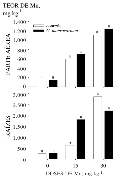
Figura 3. Teor de Mn na parte aérea e raízes de plantas de soja colonizadas por Glomus macrocarpum e plantas-controle, na média dos cultivares IAC-13 e IAC-31 Foscarin, em cada dose de Mn adicionada ao substrato. Letras iguais, na mesma dose de Mn, não diferem entre si (Tukey P < 0,05).
