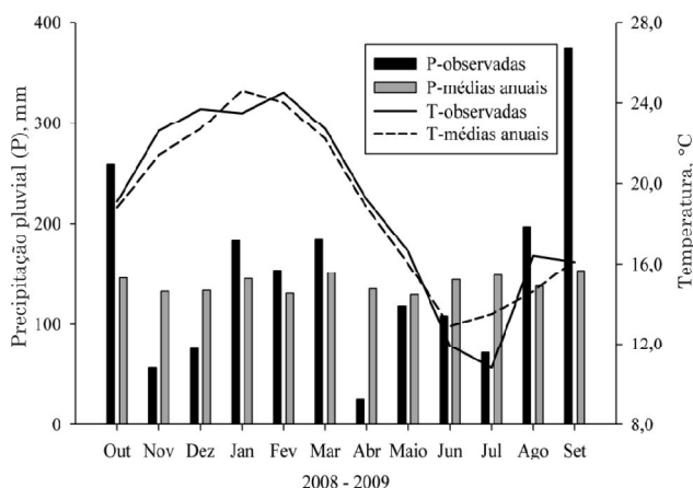
Figura 1. Precipitações pluviiais (coleta in loco ) e temperaturas médias (INMET) observadas e normais para o período de outubro de 2008 a setembro de 2009, em Santa Maria, RS.
