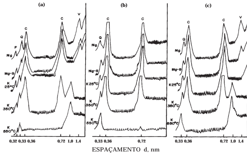
Figura 2. Difratoformas de raios-X da fração argila orientada dos tratamentos com K e aquecimento (K 25, 350 e 550°C), magnésio (Mg) e magnésio + etileno glicol (Mg + G) dos horizontes do perfil de Solonetz Solodizado: (a) horizonte A; (b) horizonte 2Btn e (c) horizonte 2CB. (C = caulinita; V = vermiculita e Q = quartzo).
