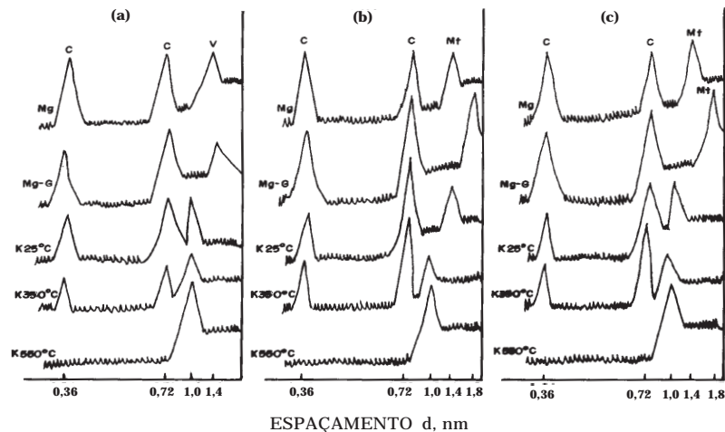
Figura 1. Difratoformas de raios-X da fração argila orientada dos tratamentos com K e aquecimento (K 25, 350 e 550°C), magnésio (Mg) e magnésio + etileno glicol (Mg + G) dos horizontes do perfil de Planossolo Solódico: (a) horizonte A; (b) horizonte 2Btn e (c) horizonte 2Cr. (C = caulinita; V = vermiculita e Mt = montmorilonita).
