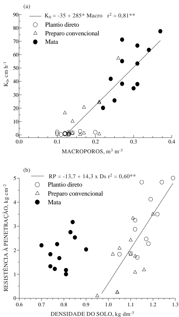
Figura 1. Relação entre a condutividade hidráulica saturada ( K_p ) e a macroporosidade para os três sistemas (a) e entre a resistência do solo à penetração e a densidade do solo nos sistemas de preparo convencional e plantio direto (b) em um Nitossolo Vermelho.
