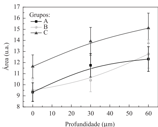
Figura 4. Áreas calculadas pela integração das bandas dos modos vibracionais na região de 887 a 1005 \text{cm}^{-1} (R3), dos grupos A, B e C. As linhas mostram as tendências em função da profundidade.
