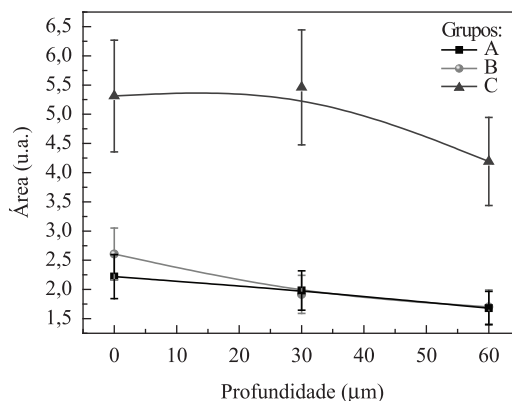
Figura 5. Áreas calculadas pela integração das bandas dos modos vibracionais na região de 1168 a 1226 \text{cm}^{-1} (R6), dos grupos A, B e C. As linhas mostram as tendências em função da profundidade.
