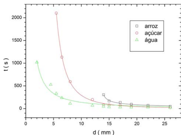
Figura 2 - Tempos de esvaziamento ( t ) de um cilindro em função do diâmetro ( d ) do furo na superfície inferior para grãos de arroz (quadrado), de açúcar (círculo) e água (triângulo). As linhas contínuas são o melhor ajuste dos dados experimentais à Eq. (1).
