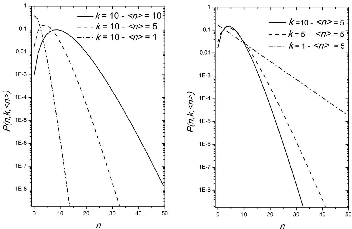
Figura 2: Gráficos da Distribuição Binomial Negativa, Eq. (36). No painel esquerdo o valor do parâmetro k é mantido constante, variando-se os valores do valor médio \langle n \rangle . No painel da direita \langle n \rangle é constante e os valores de k são alterados.
