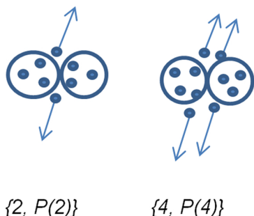
Figura 1: Ilustração da produção de partículas na colisão entre dois prótons, representados pelos círculos maiores. Círculos menores, no interior dos maiores, representam os constituintes dos prótons. As partículas produzidas na colisão são ilustradas pelos pequenos círculos com setas.
