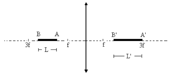
Figura 2 - Um fio retilíneo de comprimento L e extremidades A e B sobre o eixo óptico de uma lente convergente e a sua imagem.
