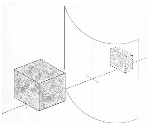
Figura 7 - Um cubo e a sua imagem virtual, menor e reversa (tronco de pirâmide) formada por meio de um espelho convexo.
