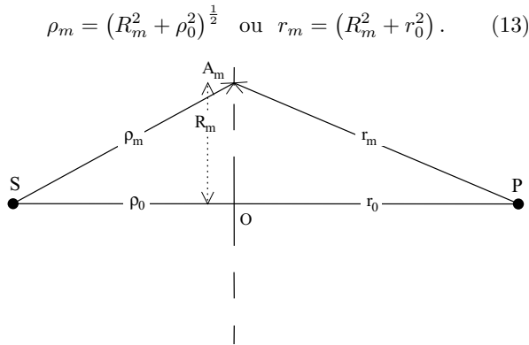
Figura 2 - Geometria da placa de zonas de Fresnel.
