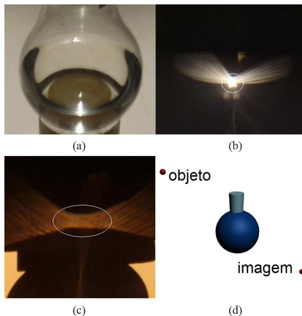
Figura 3 - (a) Um bulbo de lâmpada com água representando uma lente esférica plano-convexa. (b) A imagem de uma fonte pontual em foco fora de eixo. (c) Uma imagem difusa fora de eixo. (d) Situação geométrica do processo de imagem.
