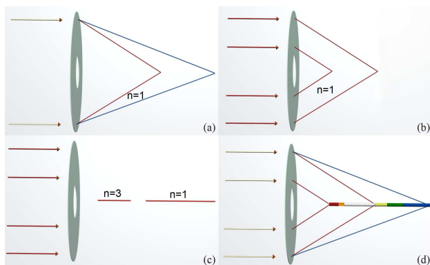
Figura 1 - (a) luz policromática vinda de um pequeno anel do disco digital (primeira ordem de difração, n = 1 ). (b) luz monocromática vinda de diferentes regiões do disco (primeira ordem de difração, n = 1 ). (c) luz monocromática vinda de todo o CD formando dois feixes não-difrativos, n = 1 e n = 3 . (d) luz policromática formando uma linha colorida emergindo do CD (todas as ordens de difração estão presentes).
