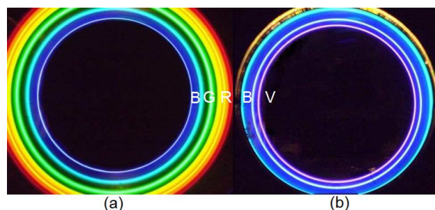
Figura 6 - (a) Câmera na posição z = (9,2 \pm 0,1) cm, as linhas espectrais da fonte B (azul), G (verde) e R (vermelho) são observadas. (b) Câmera na posição z = (21,5 \pm 0,1) cm, as linhas espectrais da fonte B (azul) e V (violeta) são observadas.
