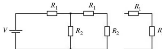
Figura 1 - Esquema de uma rede de distribuição de energia eléctrica.
