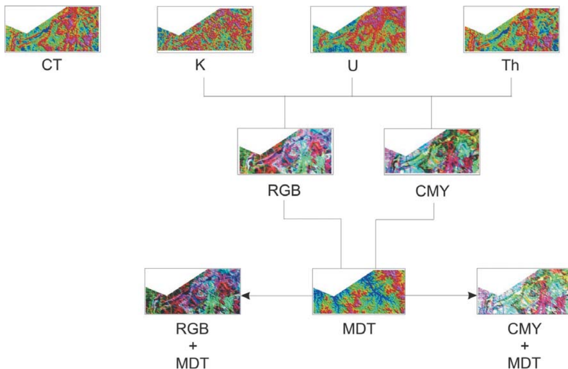
Figura 4 – Etapas de processamento dos dados gamaespectrométricos gerados para este projeto. CT – Contagem Total ( \mu R/h ), K – Canal de Potássio (%), U – Canal de Urânio (ppm), Th – Canal de Tório (ppm), RGB – Composição em falsa-cor RGB, colorida com cores aditivas primárias (Red - vermelho, Green – verde, Blue – Azul), CMY Composição em falsa-cor CMY, colorida com cores secundárias (Cian – ciano, Magenta – magenta, Yellow – amarelo). MDT – Modelo digital de terreno.
