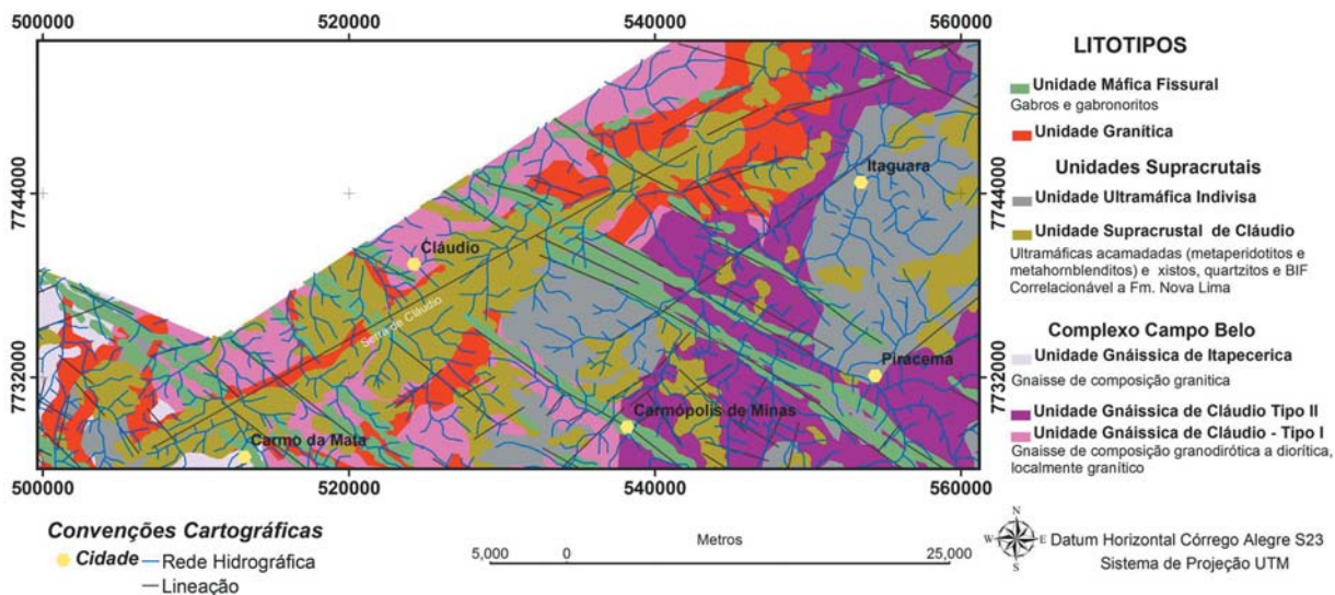
Figura 12 – Mapa Geológico confeccionado em escala 1:100.000 e apresentado em escala 1:250000. Observe que o dado destaca regiões com diferentes amplitudes na Serra de Cláudio, bem como diferencia porções do embasamento granito-gnáissico.
