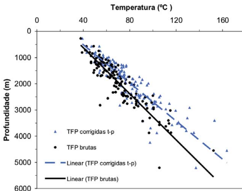
Figura 4 – Gráficos das TFPs com um único registro por profundidade corrigidas pelo esquema de tempo-profundidade (▲) e das temperaturas não-corrigidas (●), ambos em função da profundidade. Um ajuste pelos mínimos quadrados produziu um gradiente geotérmico de (27,5 \pm 1,4) \times 10^{-3} \text{ } ^\circ\text{C m}^{-1} , R^2 = 0,80 , para as temperaturas corrigidas (linha interrompida) e de (22,7 \pm 1,3) \times 10^{-3} \text{ } ^\circ\text{C m}^{-1} , R^2 = 0,74 , para as não-corrigidas (linha cheia).
