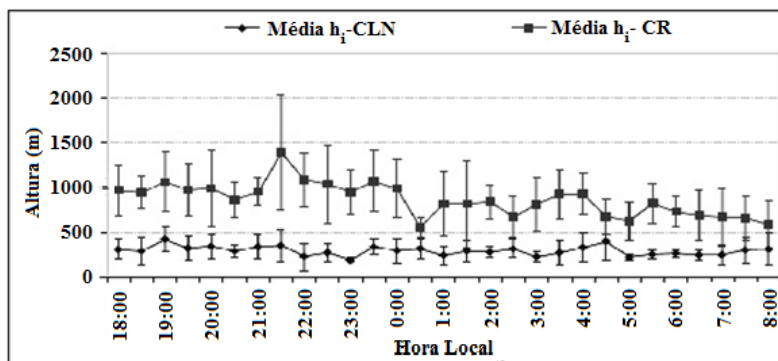
Figura 2 - Média horária das alturas da CLN e da CR obtidas com o SODAR no período de içamento do BC (20-30/10), experimento RaCCI/LBA.
