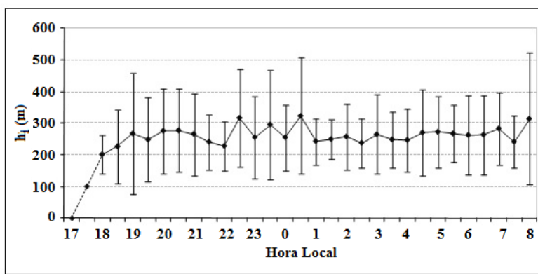
Figura 3 - Média horária das alturas da CLN com o SODAR para todo o período do experimento (06/09 à 05/11), sendo estimado o início da CLN a partir das 17 HL com a linha tracejada.
