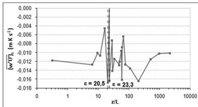
Figura 5 - Variação do fluxo de calor ( (\overline{w'\theta'})_s ) com a estabilidade ( z/L ).
