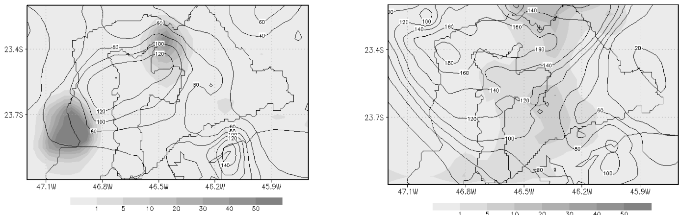
Figura 15 - Campo de precipitação (mm hora-1) e de Concentração de Ozônio (µg.m -3 ) referente ao dia 04 de março às (a)16 Z e (b) 20 Z.
