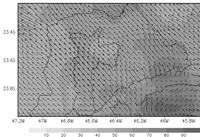
Figura 13 - Campo de Vento ( \text{m s}^{-1} ) e de Umidade Relativa do ar (%) referente ao dia 28 de fevereiro às 23 Z.
