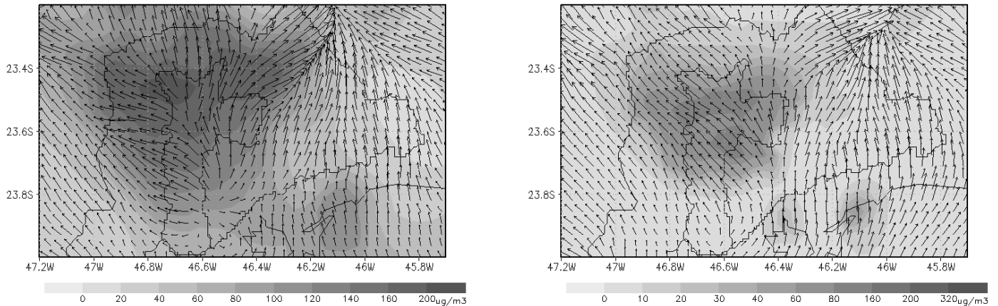
Figura 14 - Campo de Vento (m s -1 ) e de Concentração de (a) ozônio (µg.m -3 ) e (b) NO x (µg.m -3 ) referente ao dia 04 de março as 19 e 20 Z, respectivamente.
