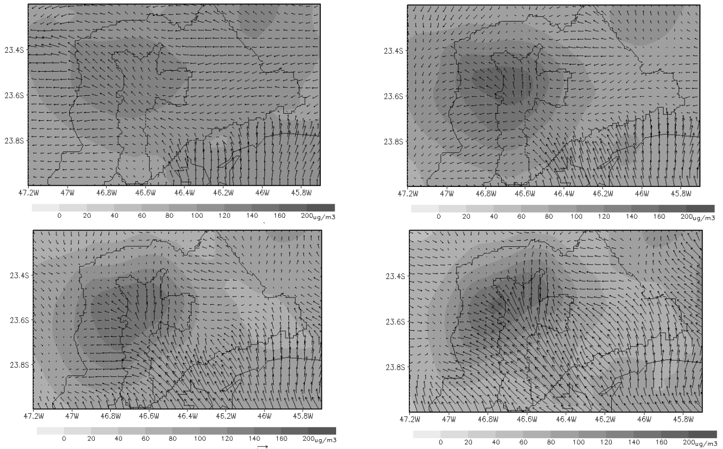
Figura 7 - Campo de Vento ( \text{m s}^{-1} ) e de Concentração de Ozônio ( \mu\text{g}\cdot\text{m}^{-3} ) referente ao dia 24 de fevereiro (a) 12 Z, (b) 14 Z, (c) 16 Z e (d) 18 Z.
