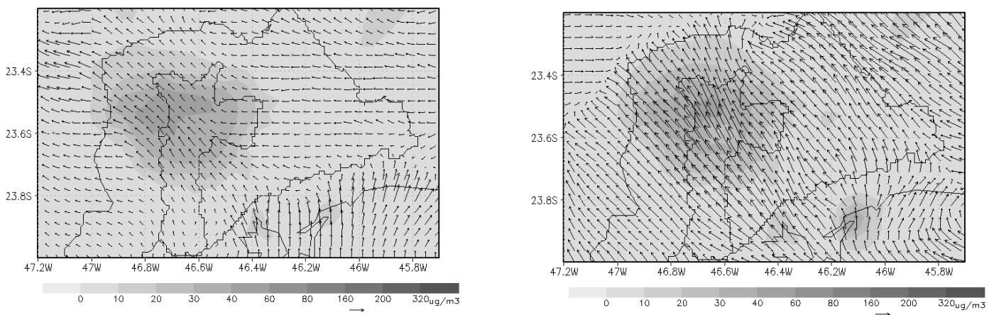
Figura 8 - Campo de Vento ( \text{m s}^{-1} ) e de Concentração de \text{NO}_x ( \mu\text{g}\cdot\text{m}^{-3} ) referente ao dia 24 de fevereiro (a) 11 Z e (b) 21 Z.
