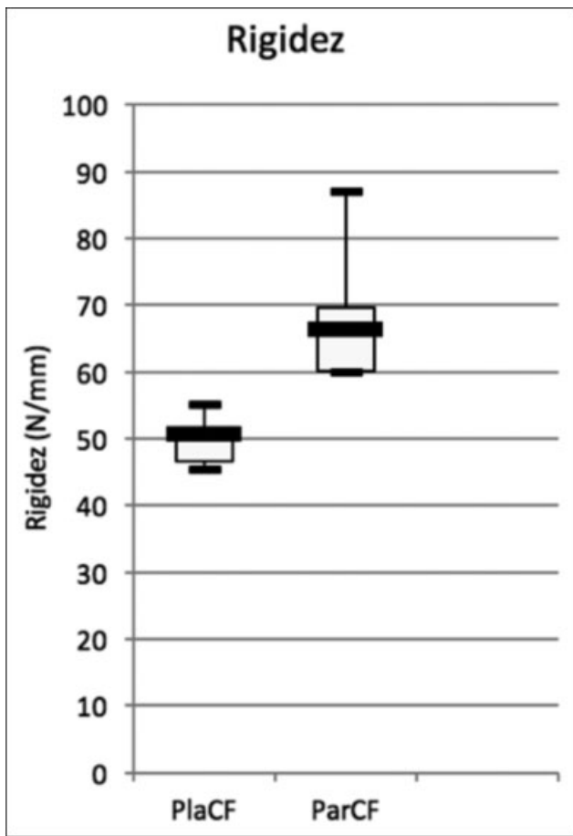
Fig. 6 Gráfico box-plot mostrando os resultados para rigidez de cada grupo testado (N/mm). O teste U de Mann-Whitney apontou significativa diferença estatística entre ParCF (dois parafusos iliossacrais em S1 fixando a articulação sacroilíaca com a sínfise púbica fixada) e PlaCF (duas placas ortogonais fixadas anteriormente à articulação sacroilíaca com a sínfise púbica fixada).
