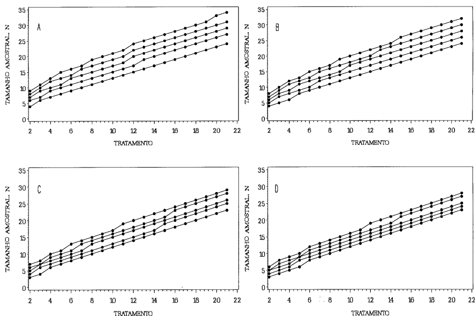
Figura 6 - Estimativas do tamanho amostral (N) para \Delta = 2,5\sigma , \alpha = 0,01 e \beta = 0,05 (A), \alpha = 0,01 e \beta = 0,10 (B), \alpha = 0,05 e \beta = 0,05 (C), \alpha = 0,05 e \beta = 0,10 (D). As linhas, em ordem decrescente de N, indicam valores acima de \rho_{\min} de 0,1; 0,3; 0,5; 0,7; e 0,9, respectivamente.
