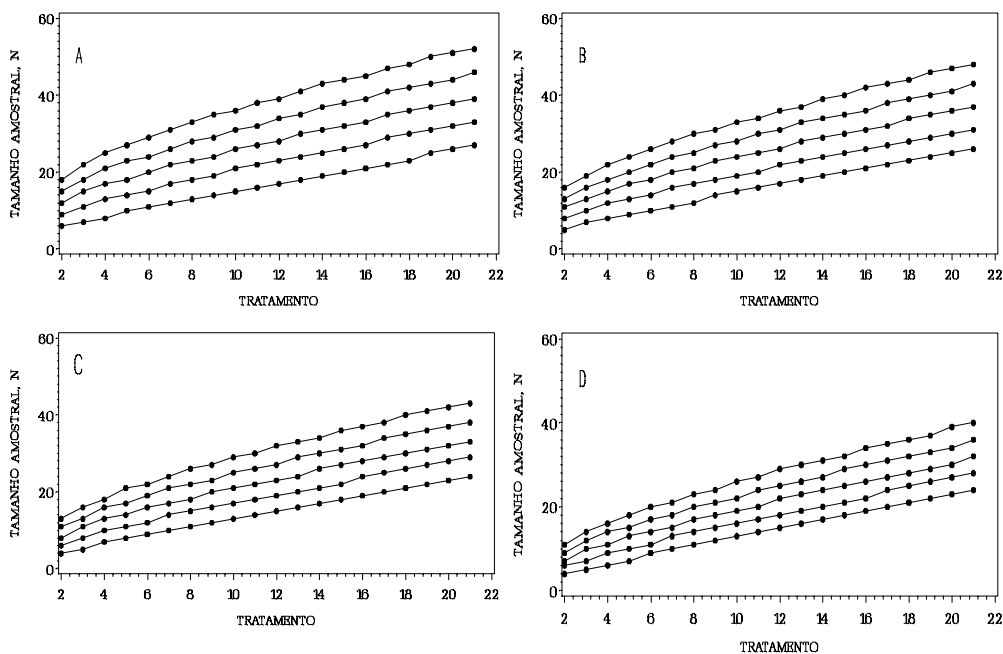
Figura 4 - Estimativas do tamanho amostral (N) para \Delta = 1,5\sigma , \alpha = 0,01 e \beta = 0,05 (A), \alpha = 0,01 e \beta = 0,10 (B), \alpha = 0,05 e \beta = 0,05 (C), \alpha = 0,05 e \beta = 0,10 (D). As linhas, em ordem decrescente de N, indicam valores acima de \rho_{min} de 0,1; 0,3; 0,5; 0,7; e 0,9, respectivamente.
