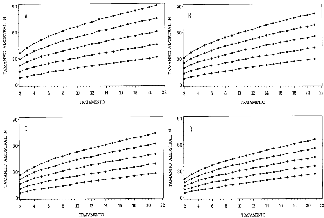
Figura 3 - Estimativas do tamanho amostral (N) para \Delta = 1,0\sigma , \alpha = 0,01 e \beta = 0,05 (A), \alpha = 0,01 e \beta = 0,10 (B), \alpha = 0,05 e \beta = 0,05 (C), \alpha = 0,05 e \beta = 0,10 (D). As linhas, em ordem decrescente de N, indicam valores acima de \rho_{min} de 0,1; 0,3; 0,5; 0,7; e 0,9, respectivamente.
