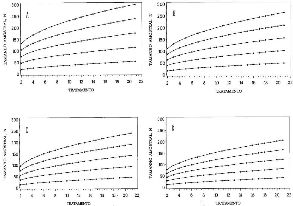
Figura 2 - Estimativas do tamanho amostral (N) para \Delta = 0,5\sigma , \alpha = 0,01 e \beta = 0,05 (A), \alpha = 0,01 e \beta = 0,10 (B), \alpha = 0,05 e \beta = 0,05 (C), \alpha = 0,05 e \beta = 0,10 (D). As linhas, em ordem decrescente de N, indicam valores acima de \rho_{min} de 0,1; 0,3; 0,5; 0,7; e 0,9, respectivamente.
