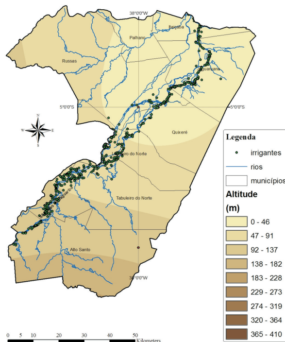
Figura 2 - Altitude (m) da área de estudo
