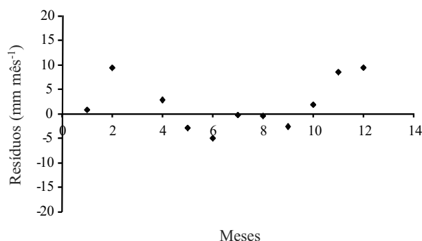
Figura 5 - Resíduos da regressão linear da E_{t_{os}} (mm mês -1 ) estimada com dados da normal climatológica e dados do modelo PRECIS HadRM3P (1961-1990)
