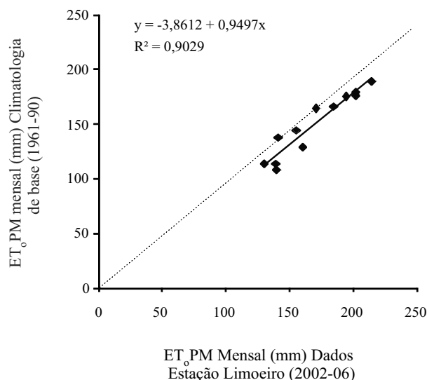
Figura 6 - Regressão linear da Et_0 (mm mês -1 ) estimada com conjunto completo de dados medidos (2002-2006) e hindcasts do modelo de mudanças climáticas (1961-1990)
