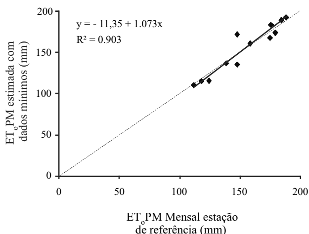
Figura 1 - Regressão linear entre E_{t_0}PM estimada com dados da estação de referência localizada em Limoeiro do Norte-CE e com dados limitados utilizando K_R=0,17
