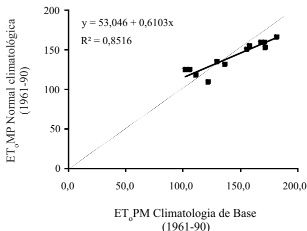
Figura 4 - Regressão linear entre a E_{t_{os}} (mm mês -1 ) estimada com dados da normal climatológica e com dados de referência (baseline) do modelo PRECIS HadRM3P (1961-1990)
