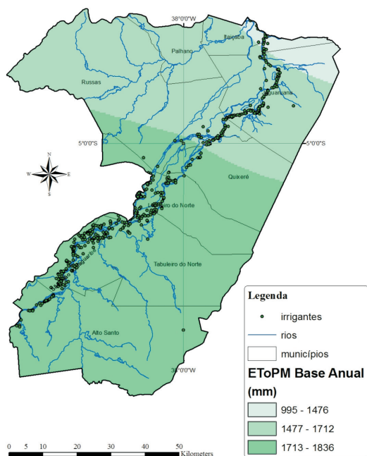
Figura 3 - Mapa temático da E_t PM anual média (mm) para o período de 1961-1990
