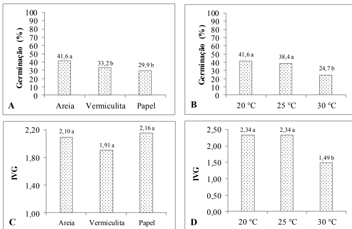
Figura 3. Germinação (A e B) e índice de velocidade de germinação (IVG) (C e D) de sementes de Albizia edwallii em diferentes temperaturas e substratos.
