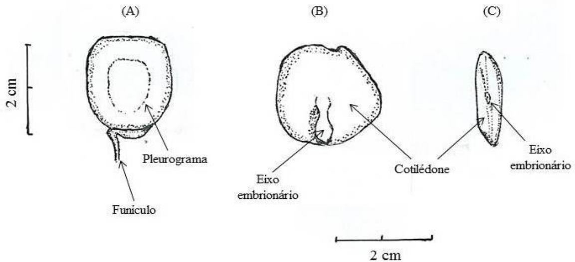
Figura 1. Morfologia externa e interna da semente de Albizia edwallii . (A) morfologia externa; (B) morfologia interna; (C) corte transversal.
