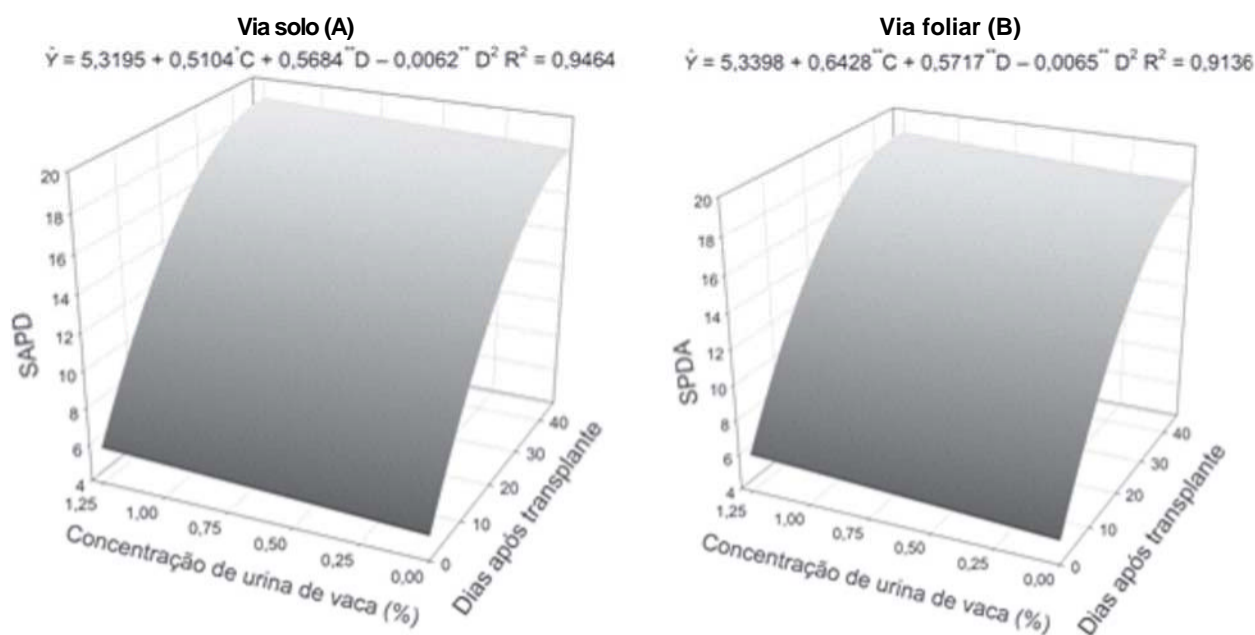
Figura 1 - Estimativa da leitura SPAD em razão da concentração de soluções de urina de vaca (C) e de dias após o transplante (D) aplicadas vias solo (A) e foliar (B) em alface 'Regina 2000'. ** e *: Significativo, respectivamente, a 1 e 5% de probabilidade.
