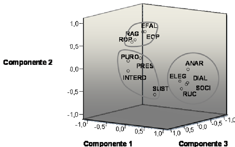
Gráfico 2 – Componentes Principais.
