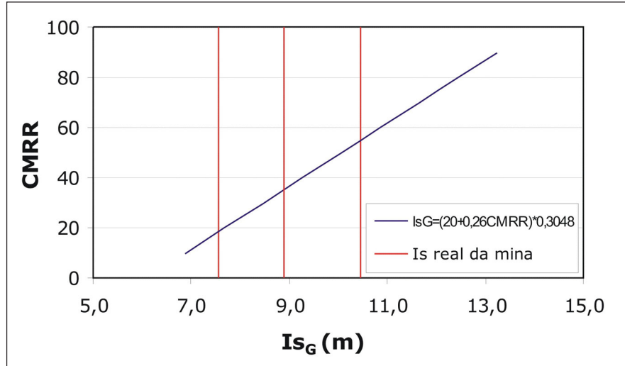
Figura 2 - Largura da diagonal nos cruzamentos das galerias. As linhas verticais representam as larguras 7,55m, 8,89m e 10,45m.
