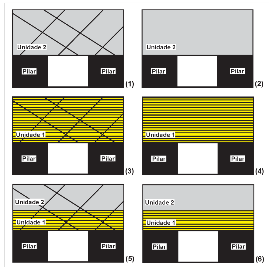
Figura 1 - Cenários de teto imediato na Mina Barro Branco.
