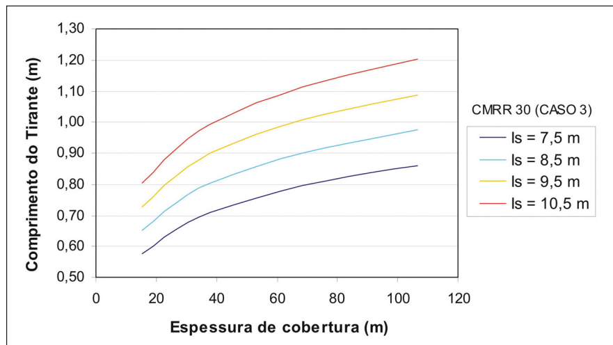
Figura 3 - Comprimento dos parafusos para a pior situação em diversas larguras de interseções (Caso 3).
