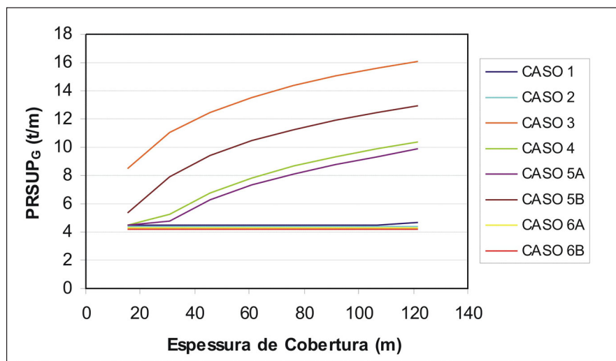
Figura 4 - Capacidade de suporte requerida.
