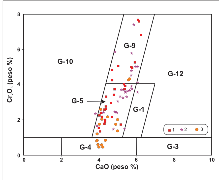
Figura 4 - Mineraloquímica CaO versus Cr 2 O 3 de granadas piropo da intrusão Abel Régis. Colorações ( 1 ) Vermelha, (*2) Púrpura e (?3) Laranja.
