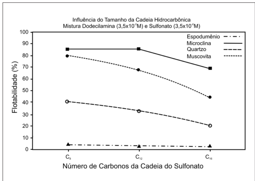
Figura 5 - Influência da cadeia hidrocarbônica do sulfonato na flotabilidade dos minerais estudados.
