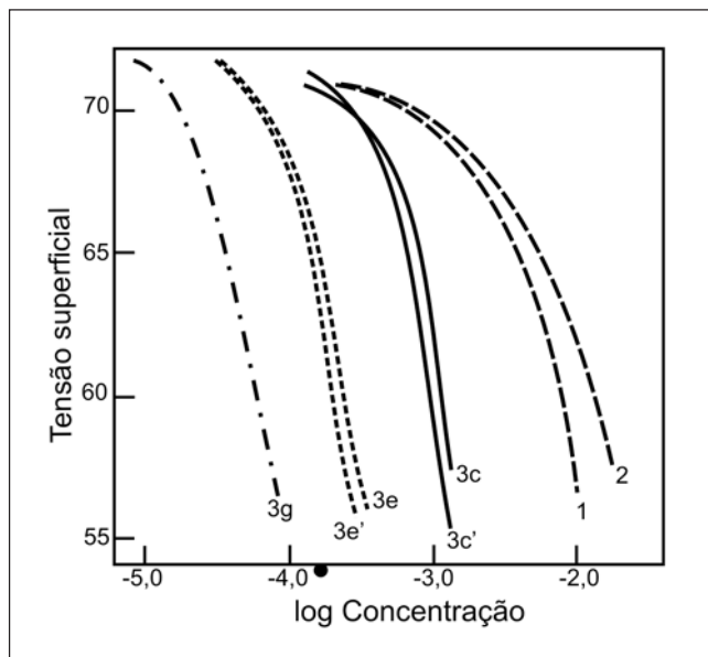
Figura 1 - Efeito sobre a tensão superficial da mistura de surfatantes aniônico e catiônico e tensão superficial da interface líquido/ar. (1) R_{10}SO_3Na , (2) R_{10}P_yCl , (3) R_{10}SO_3Na + R_{10}P_yCl : c = 1/100 , c' = 100/1 , e = 1/10 , e' = 10/1 , g = 1/1 .
