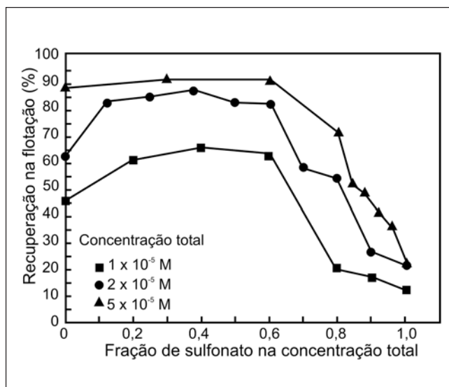
Figura 2 - Sulfonato na flotação catiônica de feldspato.
