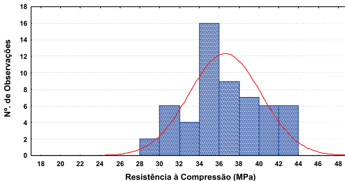
Figura 4 - Histograma dos resultados de resistência à compressão dos corpos de prova do concreto Classe C30
