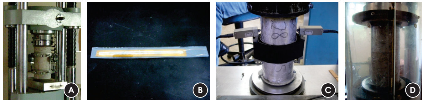
Figura 2 – Compressômetro mecânico (a) Extensômetro elétrico de colagem superficial (b), Extensômetro elétrico de fixação externa (c) e LVDT (d)
