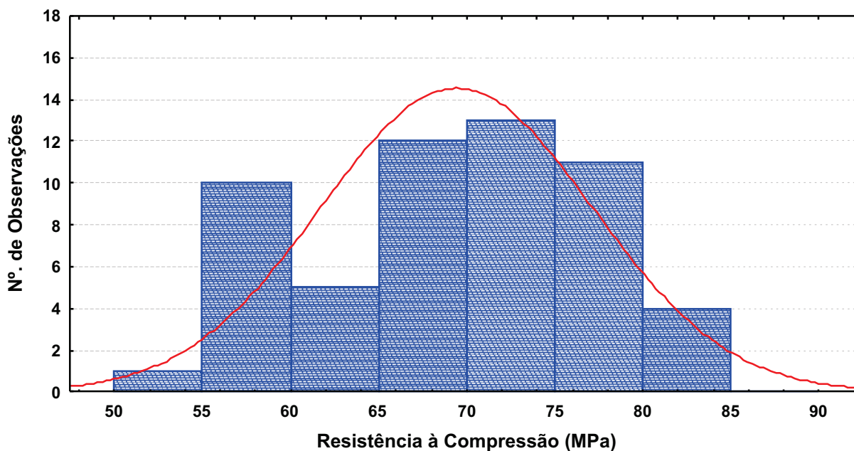
Figura 5 - Histograma dos resultados de resistência à compressão dos corpos de prova do concreto Classe C60
