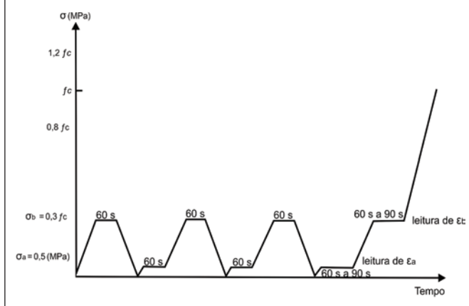
Figura 3 – Histórico do carregamento para a determinação do módulo de elasticidade – Metodologia A (ABNT NBR 8522:2008)
