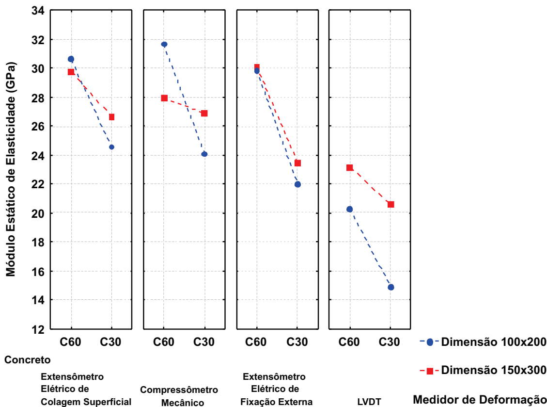
Figura 6 - Módulo estático de elasticidade, por dimensão do corpo de prova, tipo de concreto (concretos Classe C60 e Classe C30) e medidor de deformação
