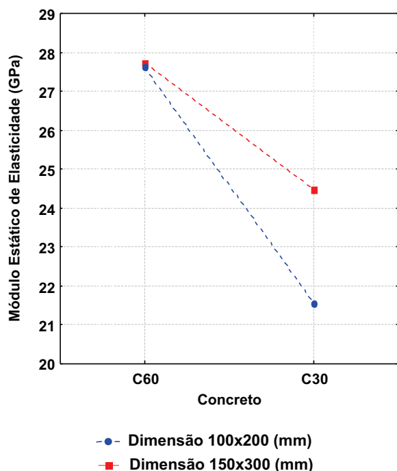
Figura 7 - Módulo de elasticidade versus tipo de concreto e dimensão do corpo de prova (inclui todos os medidores de deformação)
