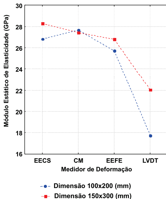
Figura 8 - Módulo de elasticidade versus o tipo de medidor de deformação e dimensão do corpo de prova (EECS - extensômetro elétrico de colagem superficial, CM - compressômetro mecânico, EEFE - extensômetro elétrico de fixação externa e LVDT)
