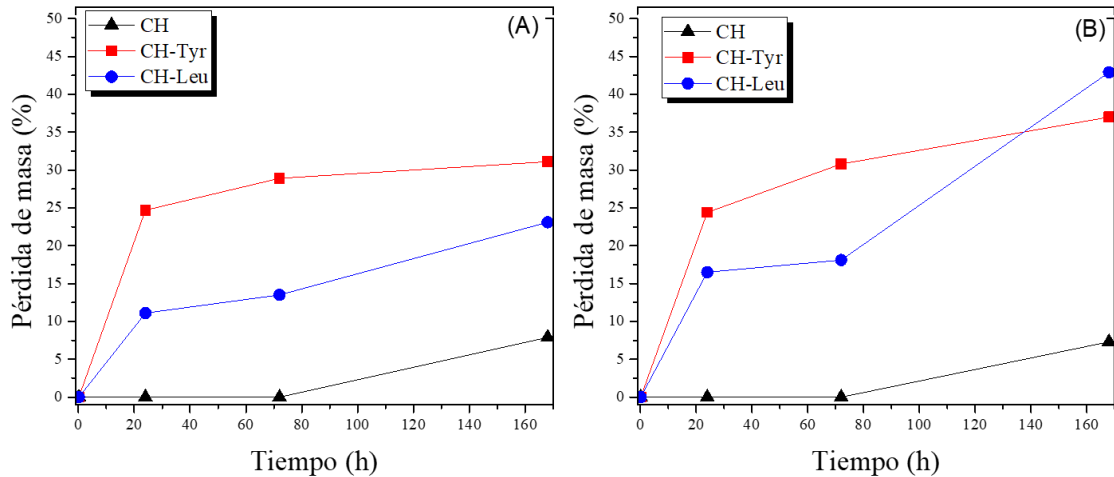
Figura 5: Evidencia del proceso de degradación por hidrólisis de las membranas de CH, CH-Tyr y CH-Leu en H 2 O destilada (pH 6,1) (A) y PBS (pH 7,4) (B) a 37°C en función del tiempo de exposición al medio hidrolítico.
