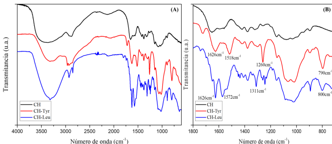
Figura 3: Espectro FTIR del CH, CH-Tyr y CH-Leu en la región de 4000-600 \text{cm}^{-1} (A) y la región de huella dactilar entre 1800-800 \text{cm}^{-1} (B).
