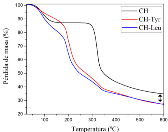
Figura 4: Termograma TGA del CH, CH-Tyr y CH-Leu
