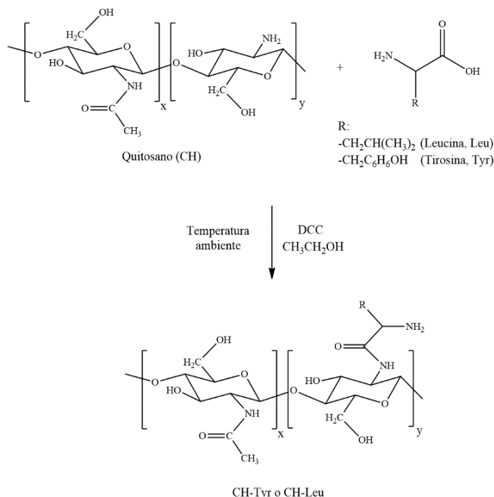
Figura 2: Reacción de quitosano con aminoácidos (Tyr o Leu) en presencia de DCC
