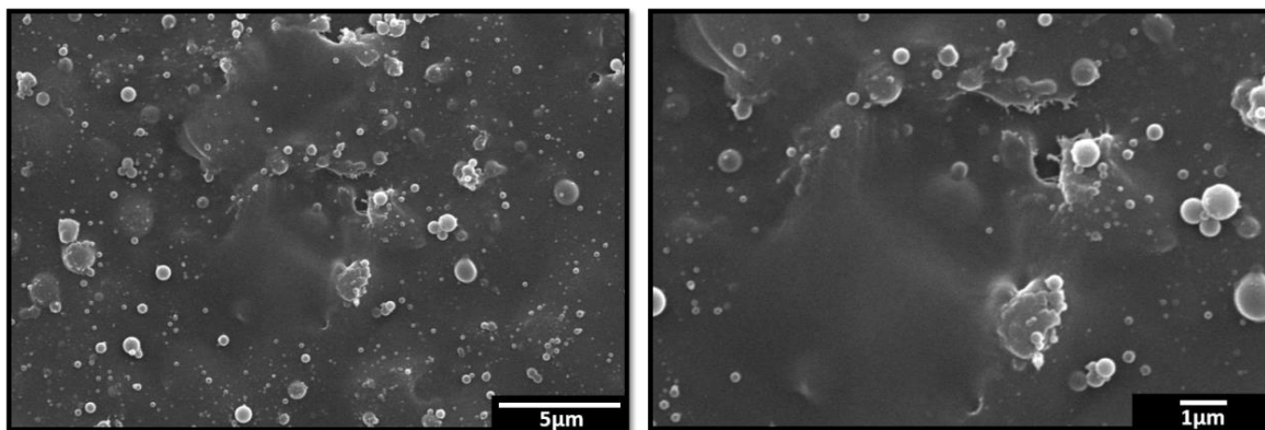
Figura 6: Microfotografía MEB (izquierda 5000X, derecha 1000X) de una solución de CH 1% (en ácido acético) donde sólo se aprecia la formación de gotas o perlas, sin evidencia de la formación de fibras (Voltaje 10 kV, distancia punta-colector de 10 cm).
