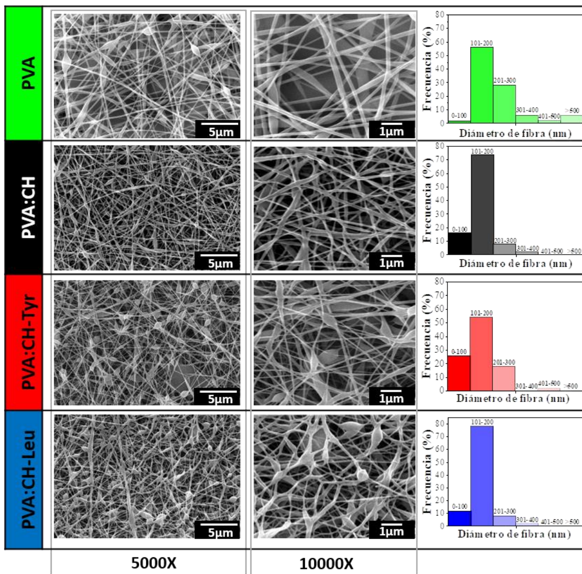
Figura 7: Micrográficas SEM (5000 y 10000 X) y gráficos de distribución de diámetro de las fibras de PVA, PVA:CH, PVA:CH-Tyr y PVA:CH-Leu.
