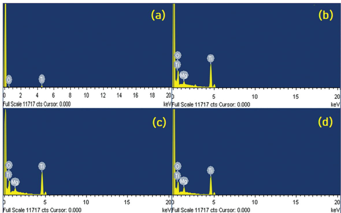
Figure 6: EDX analysis (a) MDT-1; (b) MDT-2; (c) MDT-3; (d) MDT-4.
