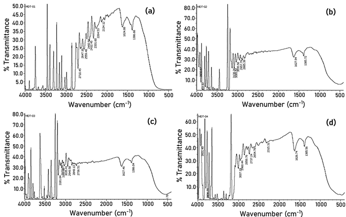
Figure 4: Infrared spectra (a) MDT-1; (b) MDT-2; (c) MDT-3; (d) MDT-4.
