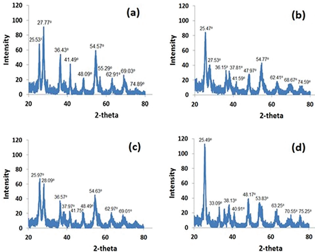
Figure 2: X-ray diffraction patterns (a) MDT-1; (b) MDT-2; (c) MDT-3; (d) MDT-4.
