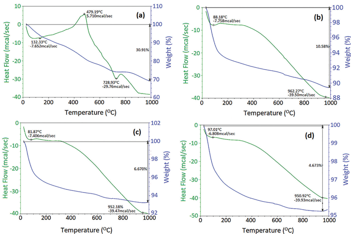
Figure 3: DSC-TGA curves (a) MDT-1; (b) MDT-2; (c) MDT-3; (d) MDT-4.
