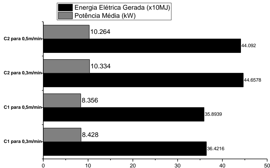
Figura 4: Potência média e energia elétrica média gerada no período de 12h para as condições C1 (PlacaQ = 950^0 C e 200 mm) e C2 (PlacaQ = 1050^0 C e 400 mm) para o projeto ‘estante’.
