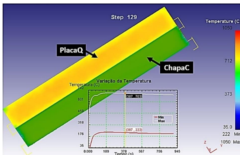
Figura 2: Exemplo de apresentação dos resultados no pós-processador do software Deform para cálculo de perfil térmico da PlacaQ do aço 1045 em contato com a ChapaC de aço inoxidável AISI 304.
