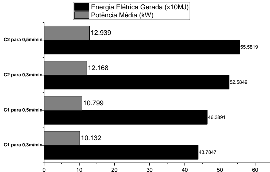
Figura 5: Potência média e energia elétrica média gerada no período de 12h para as condições C1 (PlacaQ = 950 ° C e 200 mm) e C2 (PlacaQ = 1050 ° C e 400 mm) para o projeto ‘esteira’.
