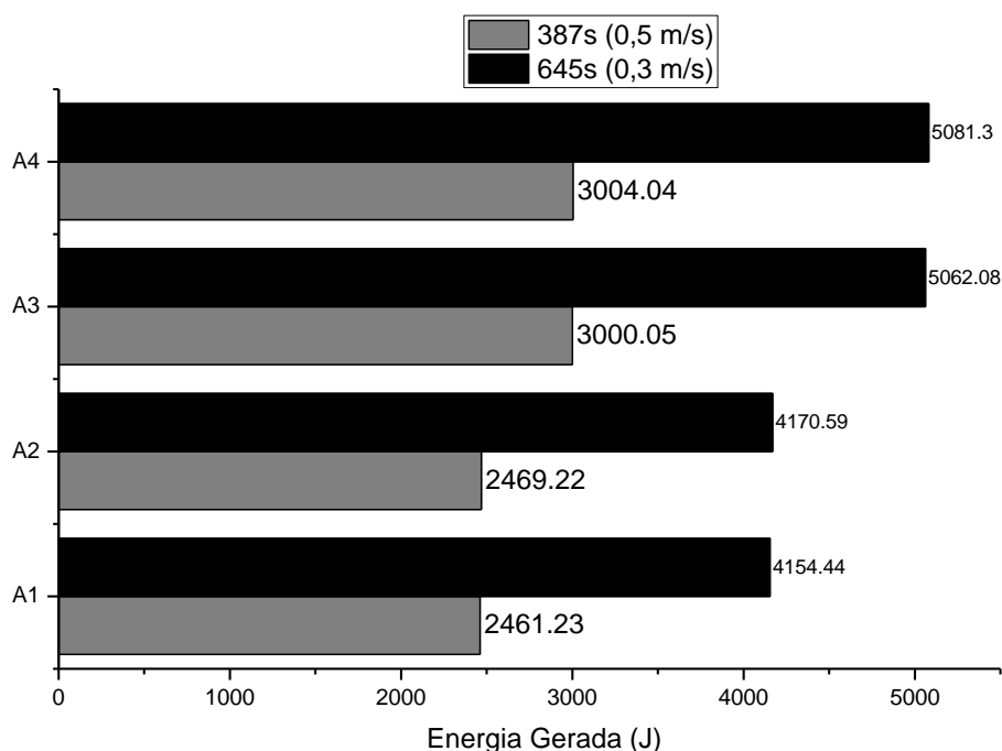
Figura 3: Comparação entre a energia elétrica gerada para as simulações A (1-4). Onde a temperatura e espessura da PlacaQ são, respectivamente: A1 - 950 o C e 200 mm; A2 - 950 o C e 400 mm; A3 - 1050 o C e 200 mm e A4 - 1050 o C e 400 mm.
