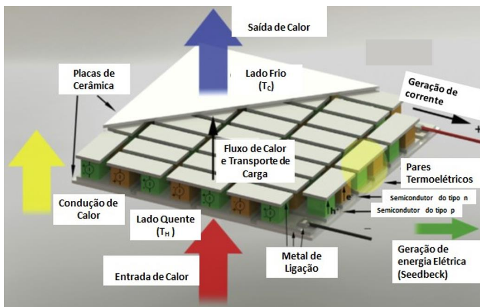
Figura 1: Modelo em 3D de um TEG e os principais efeitos físicos (adaptada de [5]).
