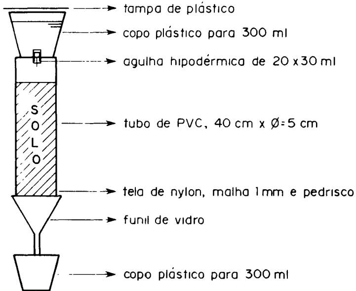
Figura 1 - Sistema utilizado para aplicação de água nas colunas e para recolhimento da solução percolada.
