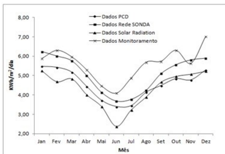
Figura 3 - Valor médio diário, por mês, de irradiação solar global extraído dos dados coletados da rede SONDA, da PCD de Ilhéus, da modelagem com uso do Solar Radiation e do monitoramento executado.
