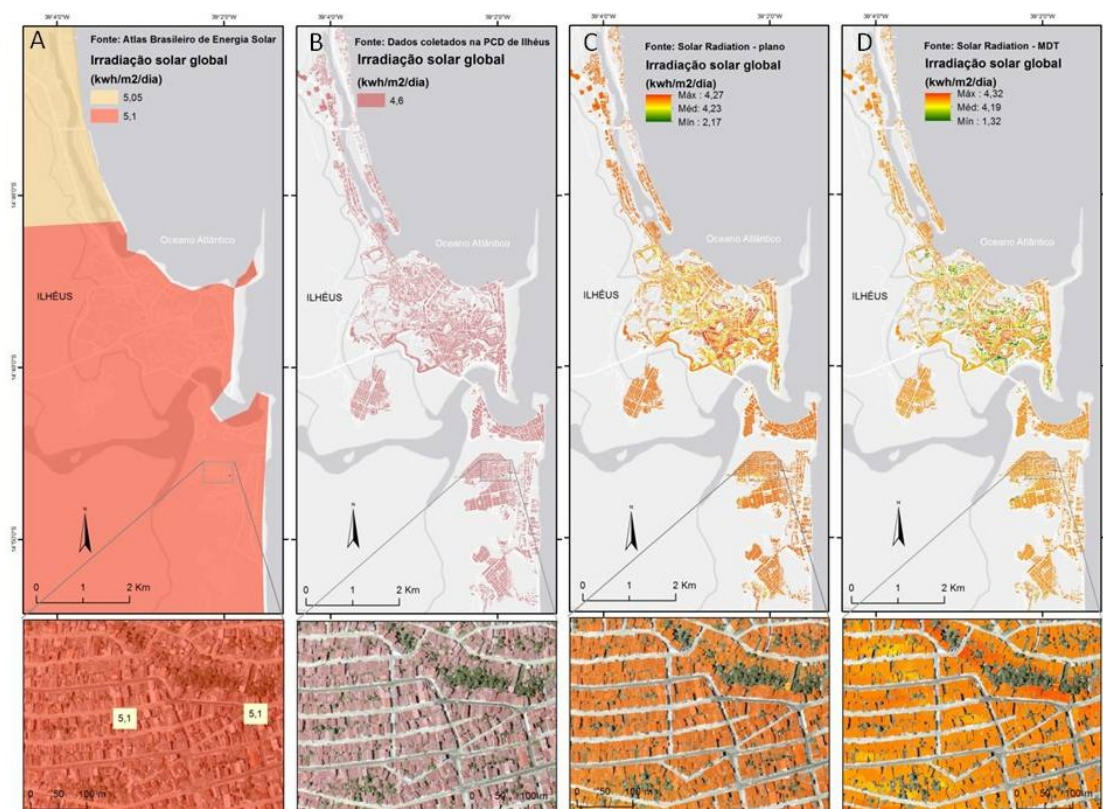
Figura 4 – Valores de irradiância solar global obtidas por diferentes métodos na área em estudo.
